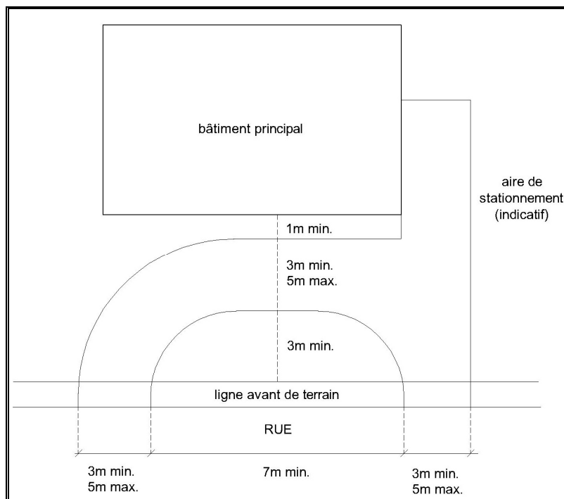
CROQUIS 29 : L'ACCÈS EN DEMI-CERCLE
