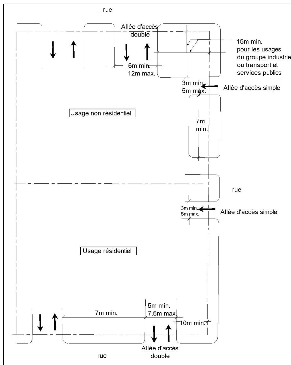
CROQUIS 28 : DISTANCE ET LARGEUR DES ALLÉES D'ACCÈS À LA PROPRIÉTÉ SIMPLE ET DOUBLE
