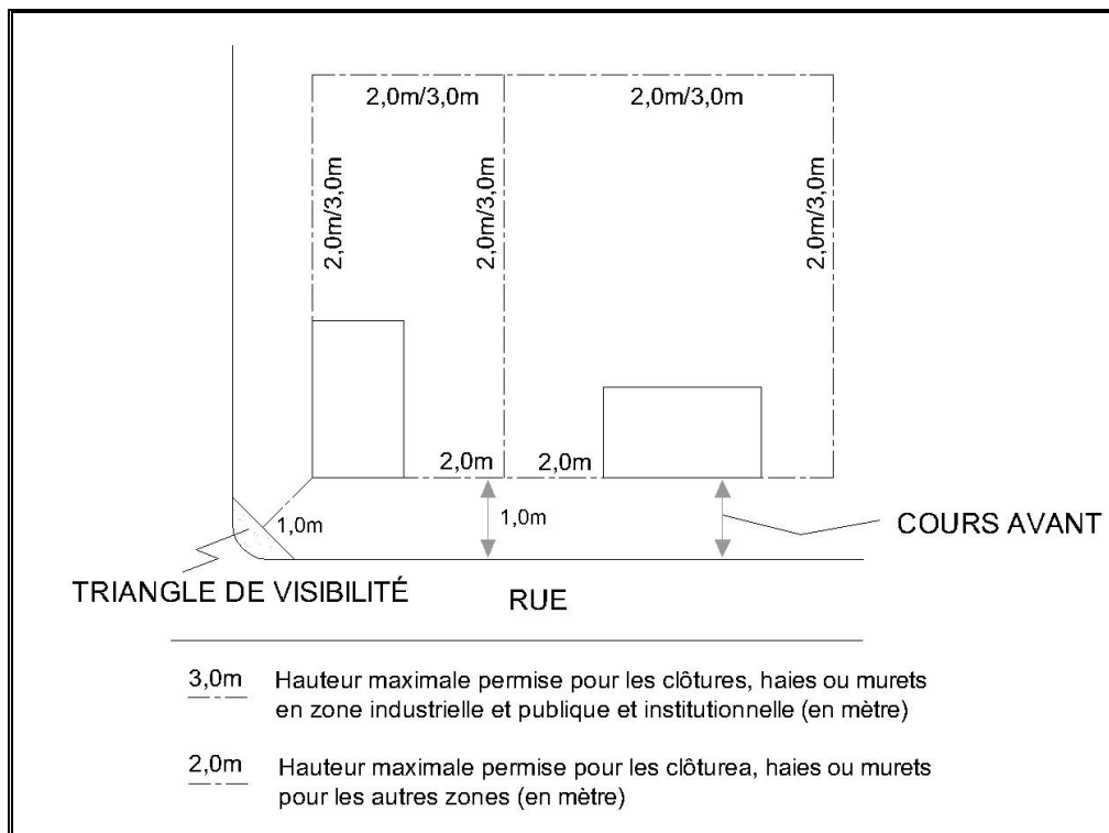
CROQUIS 26 : IMPLANTATION D'UNE CLÔTURE, D'UN MUR ET D'UNE HAIE
