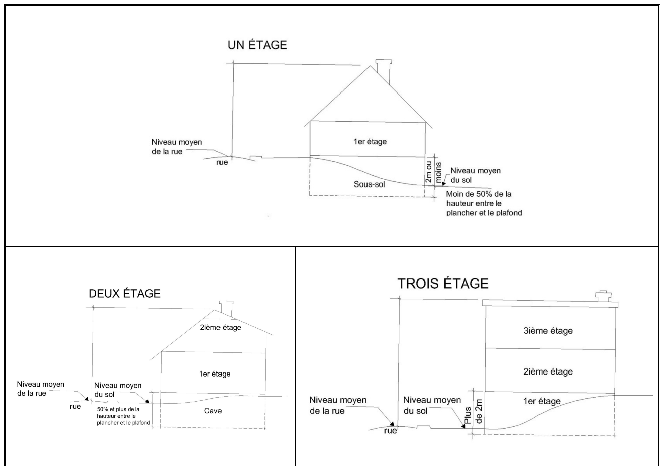
CROQUIS 7 : DETERMINATION DU NOMBRE D'ETAGE D'UN BATIMENT
