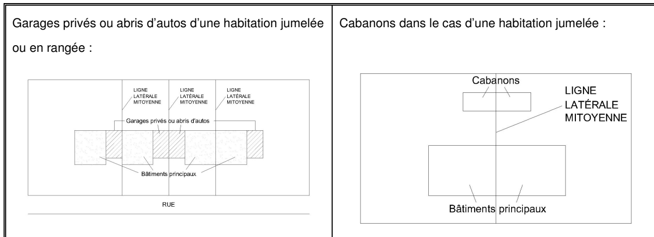
CROQUIS 24 : BÂTIMENT COMPLÉMENTAIRE À UNE HABITATION JUMELÉE OU EN RANGÉE
